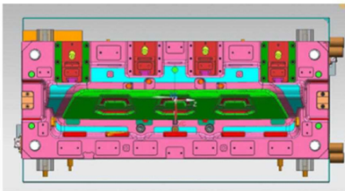
Cores
